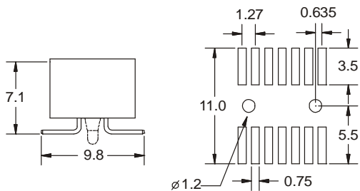
MECANIZADO RECOMENDADO
